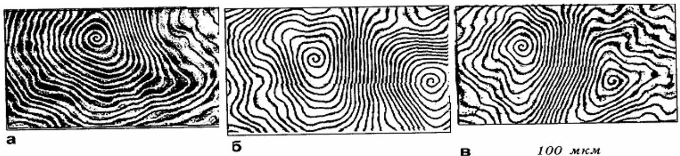
Рис.7. Спиральные динамические домены в пленке феррита-граната в переменном поле типа меандр с частотой 300 Гц и амплитудой 80 Э, сфотографированные в одном и том же месте образца последовательно с интервалом менее одной минуты (а, б, в).
