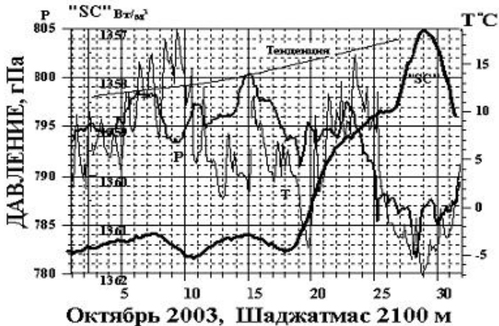
Рис.2. Изменения приземного давления P и температуры воздуха T представлены по трехчасовым данным метеостанции Шаджатмас для октября 2003 года совместно с изменениями солнечной постоянной в обращенной шкале ее значений. “Спокойный” ход синоптических вариаций в первой половине месяца нарушается в последующие недели, по-видимому, под воздействием внешнего силового фактора.
