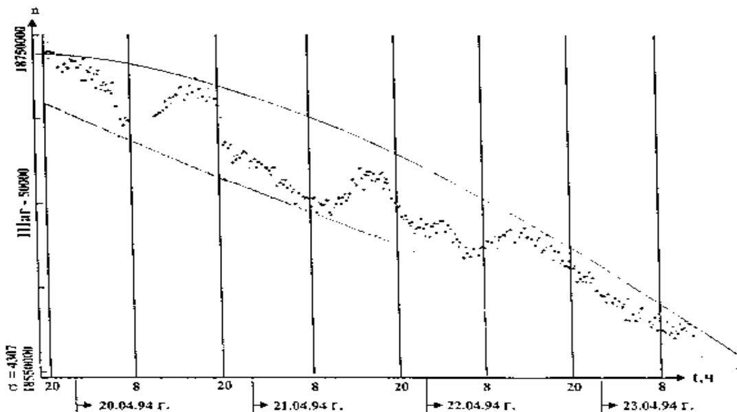
Рис.5. Вариации скорости распада церия 144. n – количество распадов за 16 минут, t – время суток (г. Санкт-Петербург, 20–23 апреля 1994 г.).
