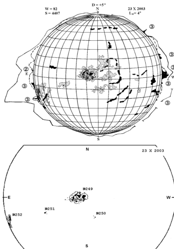
Рис.1. Гелиографическая карта магнитных полей и активных областей Солнца за 23 октября 2003 года: а – вблизи центра (немного левее) располагается мощная и компактная активная область №249. У основного пятна АО №249 площадь S=2190 мдп была максимальной именно 23.10.2003. АО №252 только появляется из-за восточного края диска Солнца, в которой 23.10. уже произошла вспышка X5.4/1B, а 24.10. – вспышка балла M7.6/1N, затем последовали мощные вспышки 26-27.10. и в завершение этой серии – сверхмощная вспышка X17.2/4B (28.10). За краем диска еще скрыта не менее мощная АО №257. Эти три АО, начиная с 18.10.2003, как раз и определяли явные вариации величины солнечной постоянно (СП) до конца октября. Темные продолговатые образования – относительно холодные волокна, удерживающие остывающую солнечную плазму в магнитных ловушках. Волнистые линии вокруг Солнца показывают равные значения яркости короны. Слева сверху указаны суммарные параметры всех расположенных на диске солнечных пятен: число Вольфа W = 82 и их площадь S = 4407 мдп (миллионных долей полусферы); б – центральная часть солнечного диска с обозначениями активных областей.
